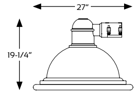
1527LED5M-R (Flat Lens)
